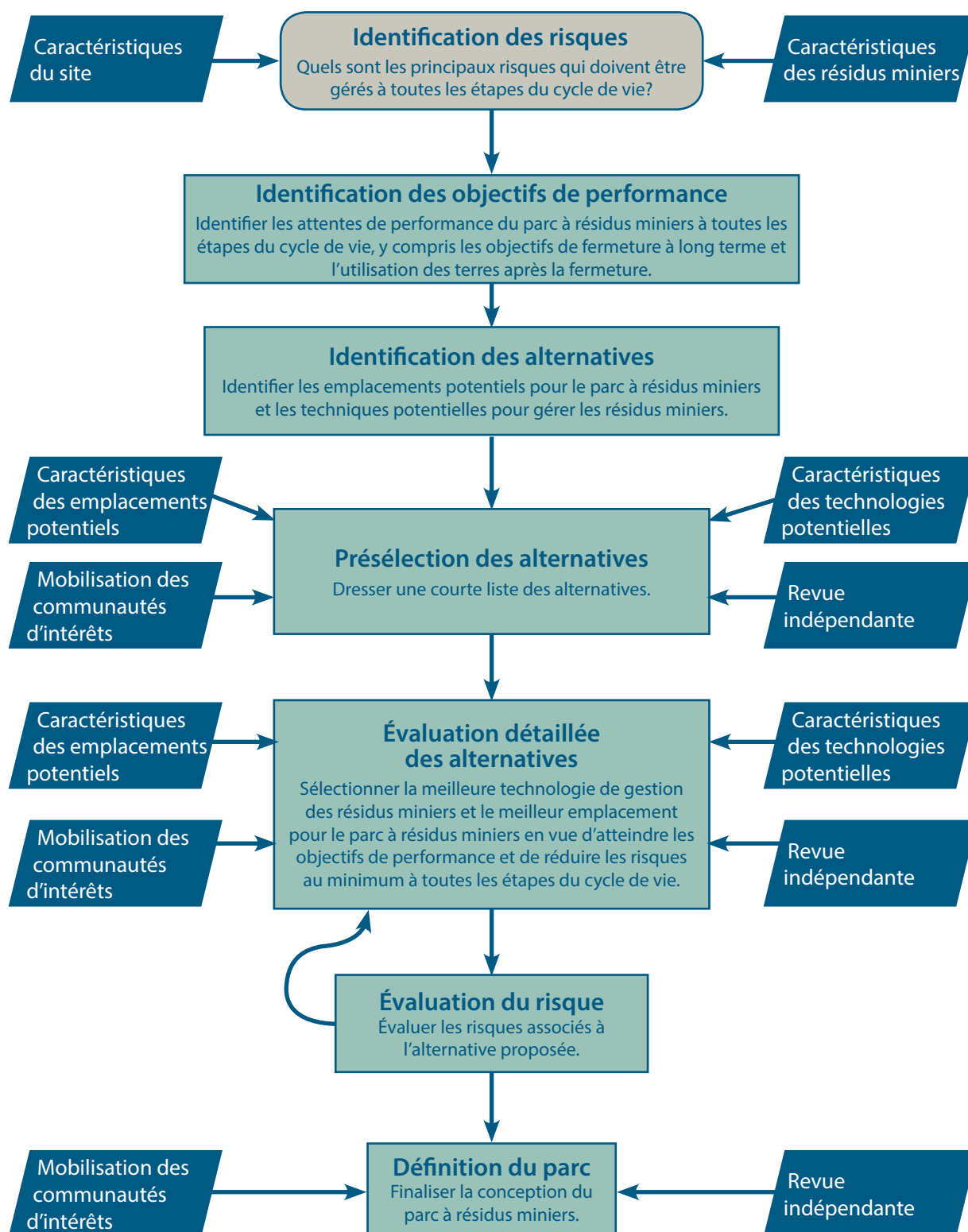
Figure A.3.1 : Cadre de planification conceptuelle des parcs à résidus miniers
